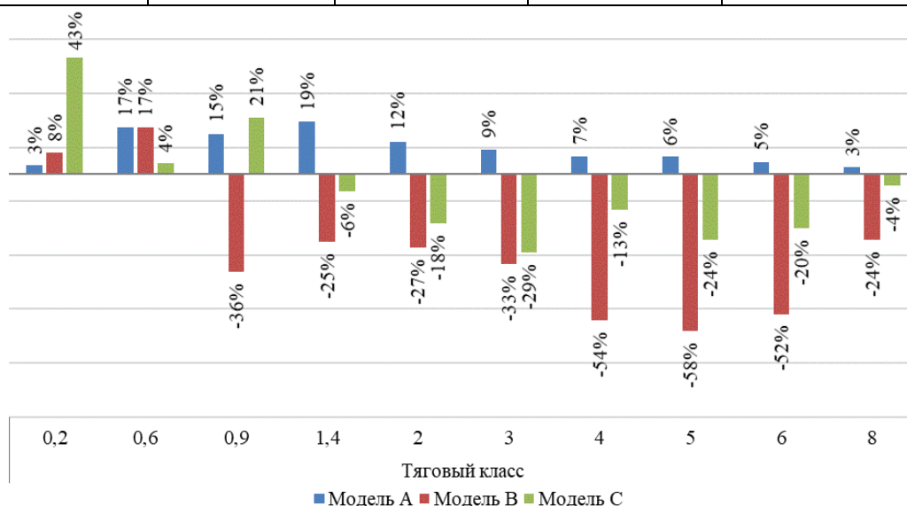
Рис. 2 – Сравнительная оценка себестоимости мото-часа работы при использовании беспилотных мобильных средств различных концептуальных моделей по отношению к базовым тракторам
