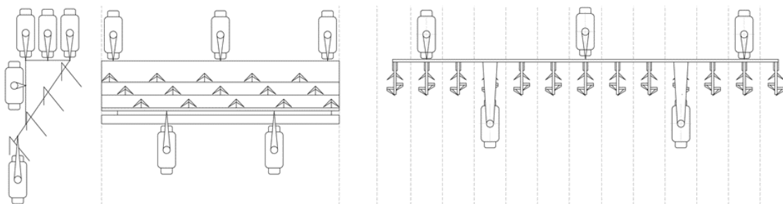
Рис. 1 – Агрегатирование беспилотных мобильных средств концептуальной модели С (энергомодулей) с плугом, культиваторами для сплошной обработки почвы и междурядной обработки пропашных культур
